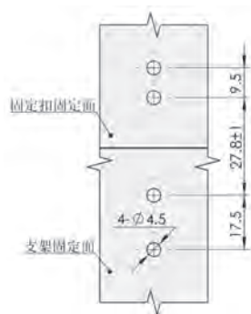
開孔尺寸 Cut Out
