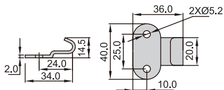
A 扣座 (TSL322-A)- 水平式安裝用
