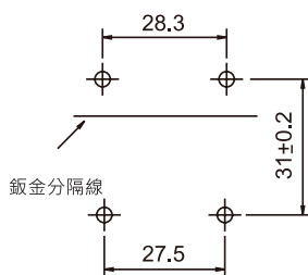
開孔尺寸 Cut Out
