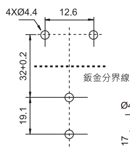
開孔尺寸 Cut Out
