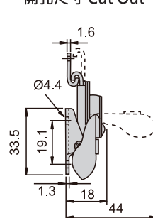
開孔尺寸 Cut Out
