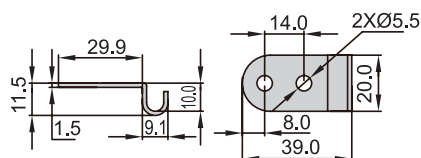
C 扣座 (TSL322-C)- 垂直式安裝用
