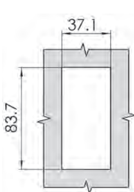
開孔尺寸 Cut Out
