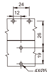
開孔尺寸 Cut Out
