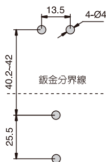
開孔尺寸 Cut Out
