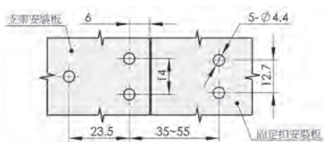
開孔尺寸 Cut Out
