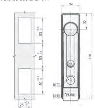
開孔尺寸 Cut Out
