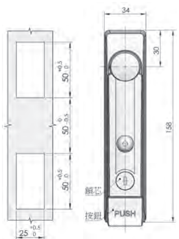
開孔尺寸 Cut Out
